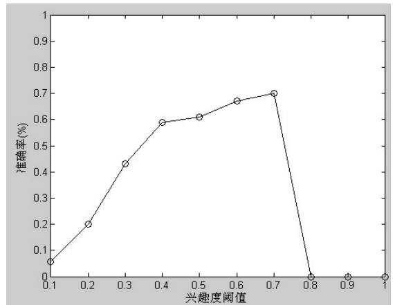
图 4 兴趣度阈值与准确率的关系
