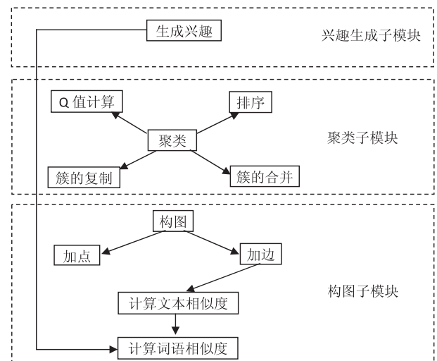
图 1 兴趣提取模块的功能结构层次图
