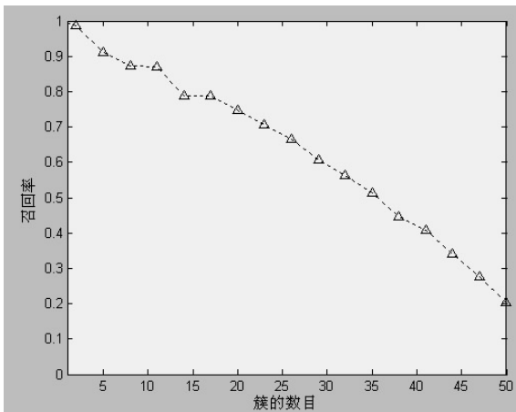
图 2 簇的数目与召回率的关系
