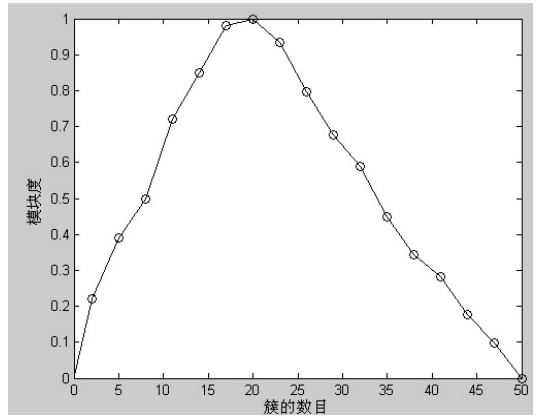
图 3 簇的数目与模块度的关系
