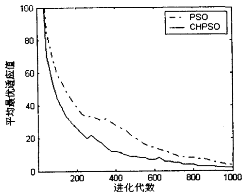
图 2 Rastrigin 函数平均最优适应值曲线
