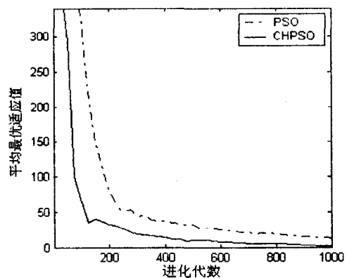
图 1 Rosenbrock 函数平均最优适应值曲线
