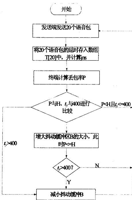
图 1 算法流程图
